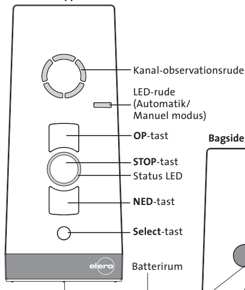
Forside af apparat
